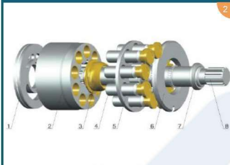
HD450V-2 KATO
