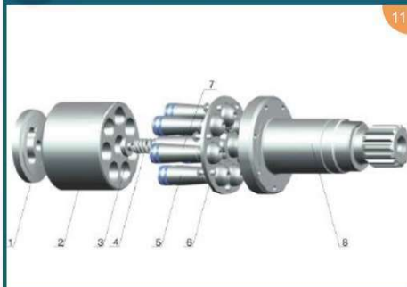
A2FO10~500
