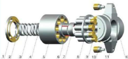
PVT38/PVT64
