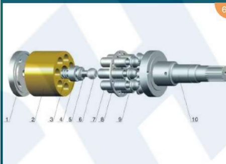
PC200-2/PC60-6
