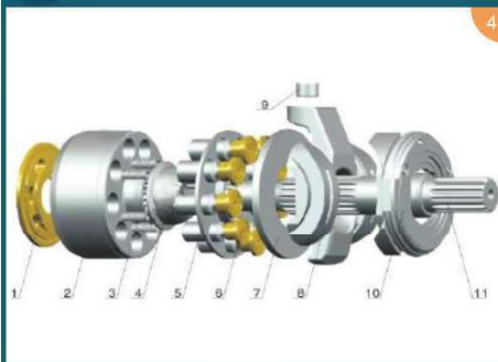
K7V63
