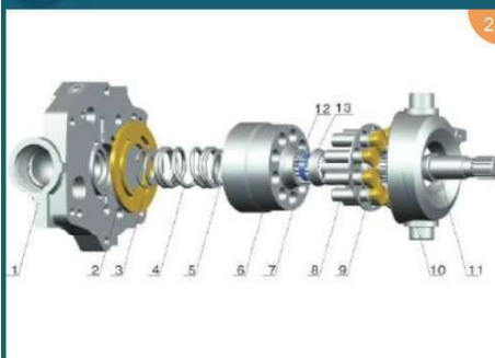
PVE19/PVE21/TA19
