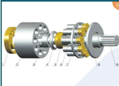
E200B/AP-12/14/SPK10/10
