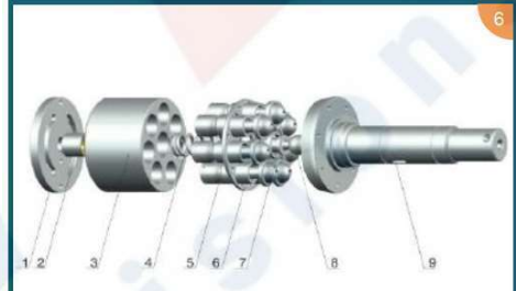
KYB33/KYB36/KYB87/KYB90(MSG-60P)
