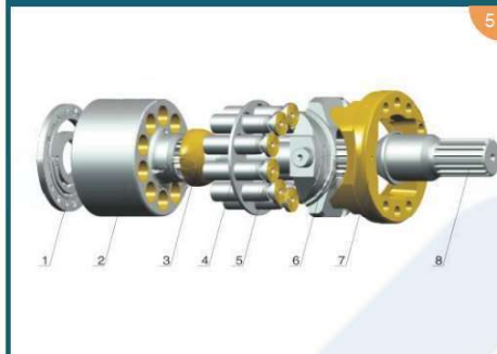
PC160
