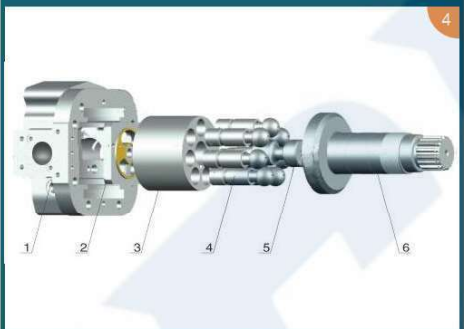
HPV116/145/125B
