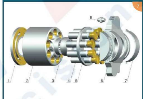
PC320
