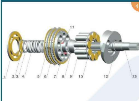
MAG150/170
