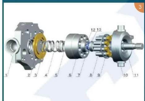
PVH45~141
