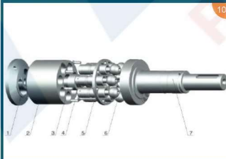
A2VK
