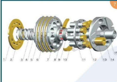
A10VSF28
