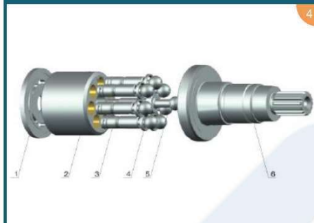
BMV75.27
