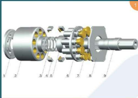
A4V40~250/A4VFO28/A4VSO40~500
