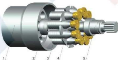
PVG130 B
