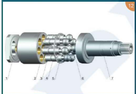
A6V28/A7V55~500
