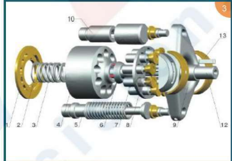
A10VSO16~45/A10VO45/52/A10VSO63~140
